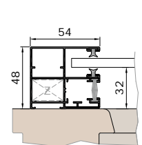
Führungsschiene KR54V
