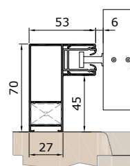
Führungsschiene ED53V
